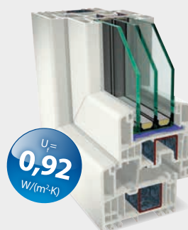
Uski okvir s krilom i ispitanom ift-pogodnosti za pasivne kuće
